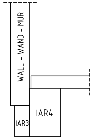
DET. B-B
