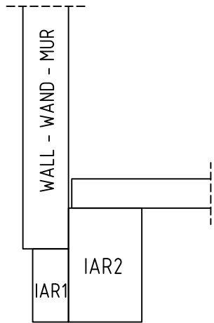
DET. A-A
