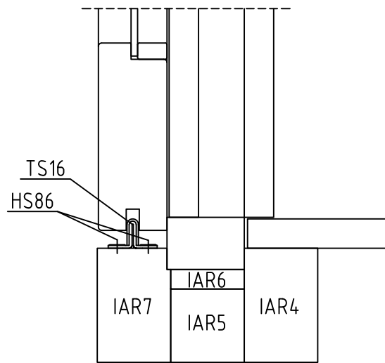
DET. D-D
