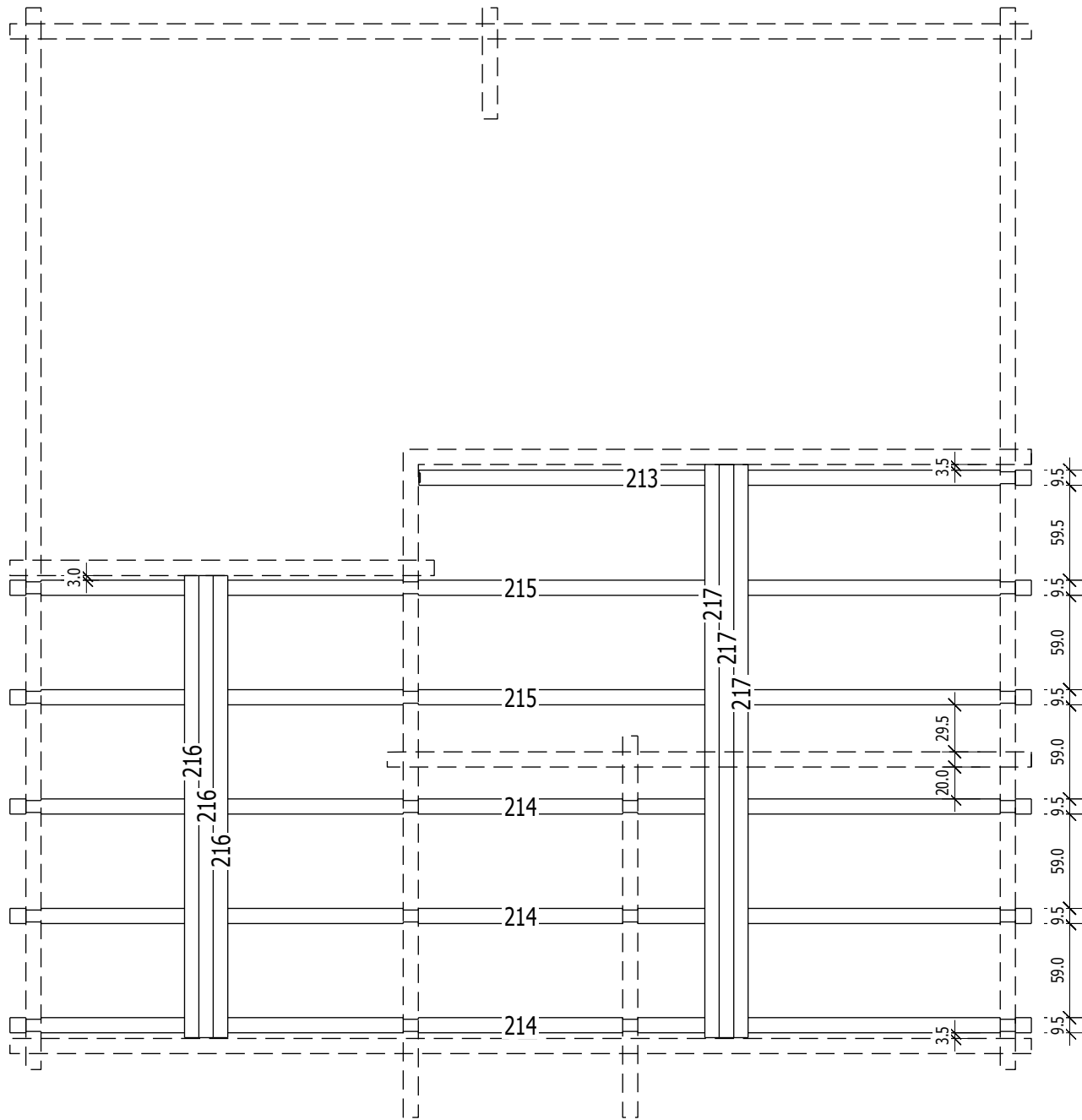
Deckenbalkenplan
