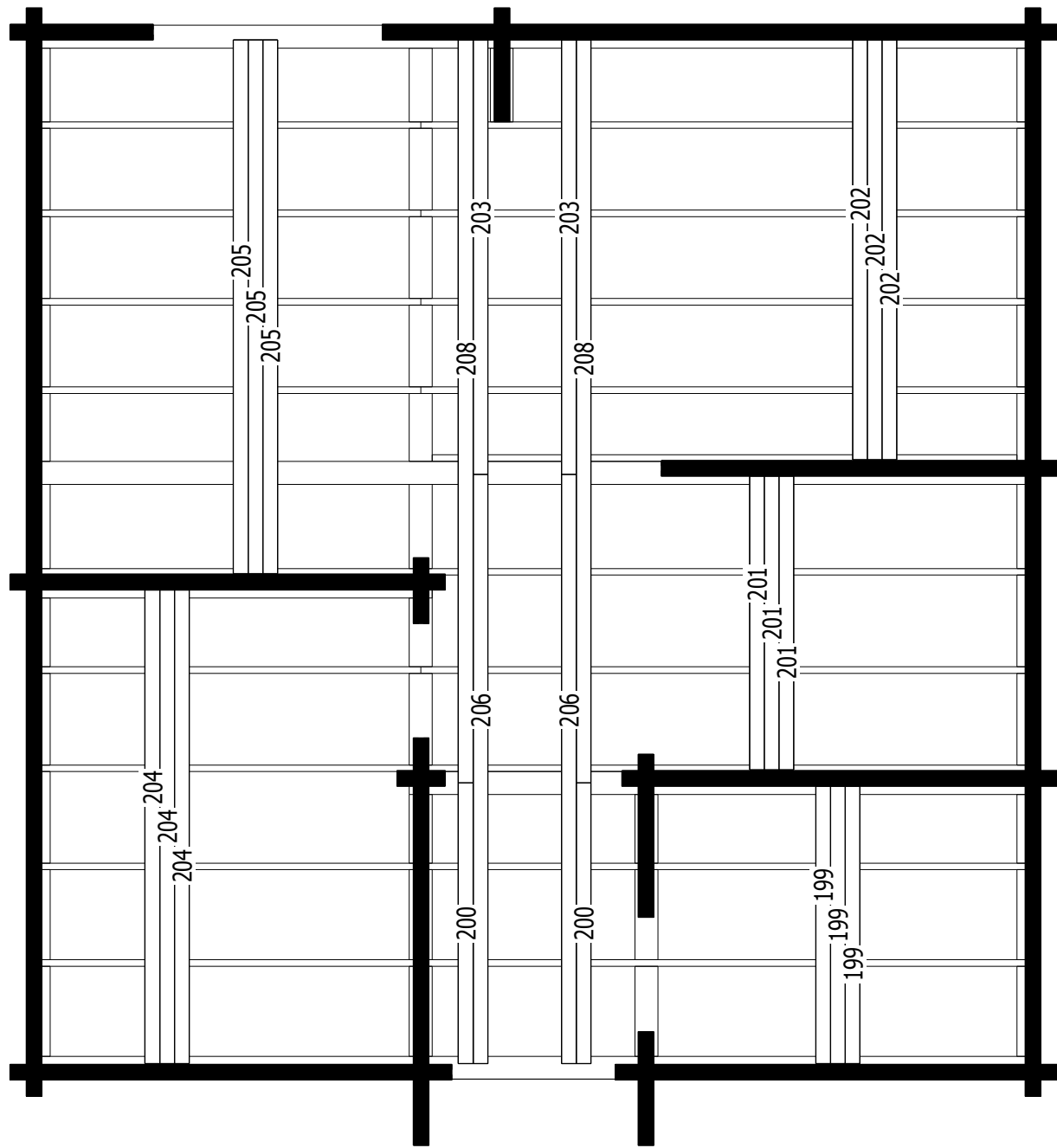
Hobeldielenplan
