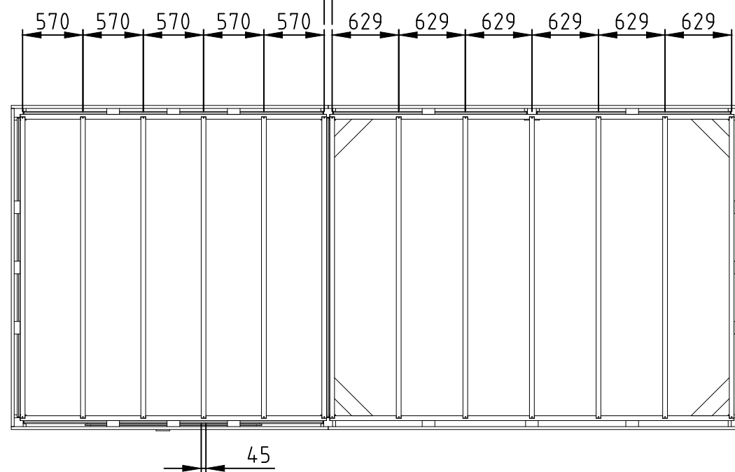
Overzicht gordingen 75
