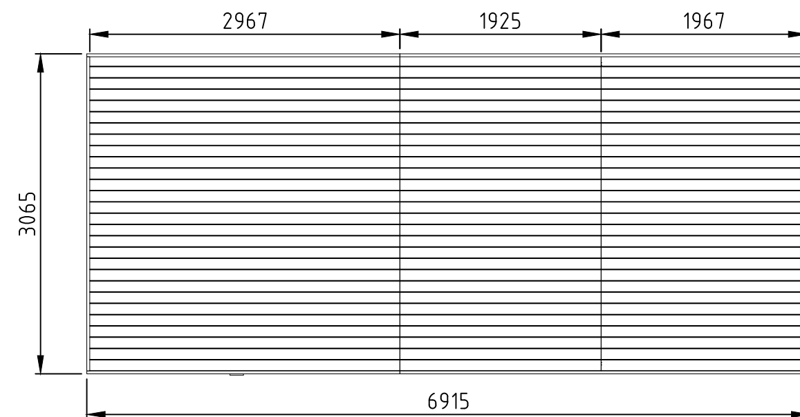
Bovenaanzicht
