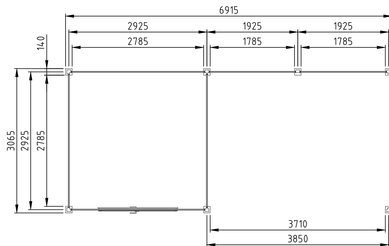
Palenplan
