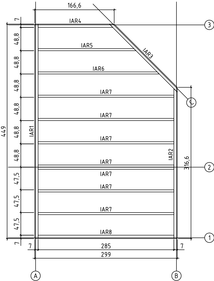
FOUNDATION - FUNDAMENT - FONDATION
