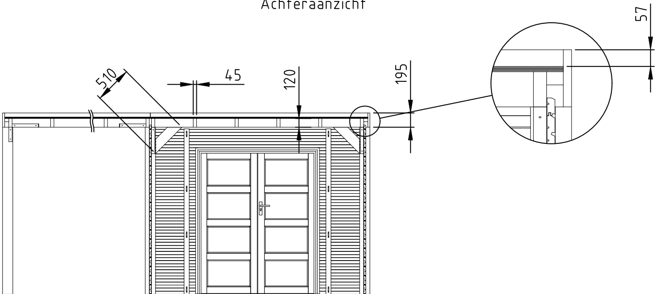
Doorsnede
