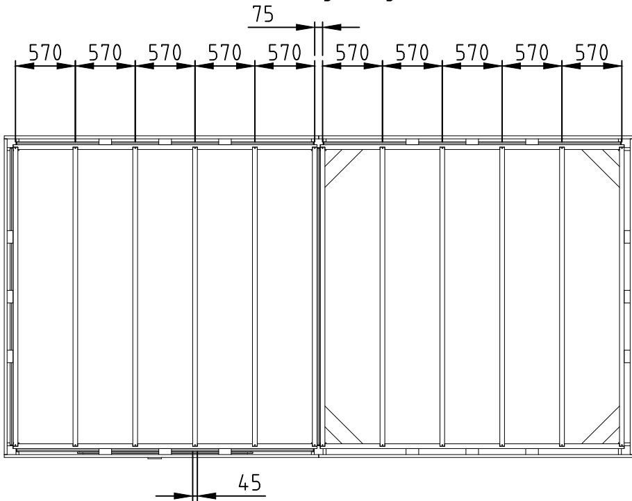
Overzicht gordingen
