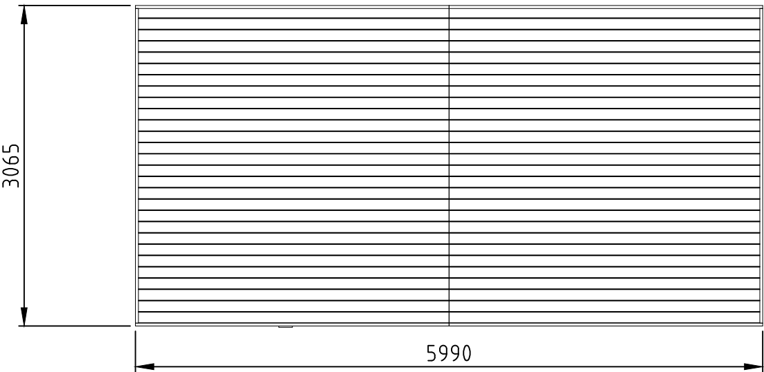
Bovenaanzicht
