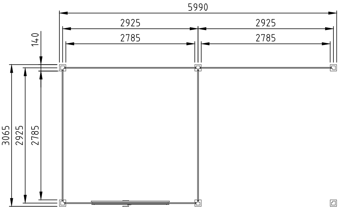
Palenplan
